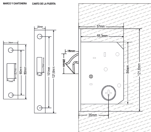
MARCO Y CANTONERA CANTO DE LA PUERTA
