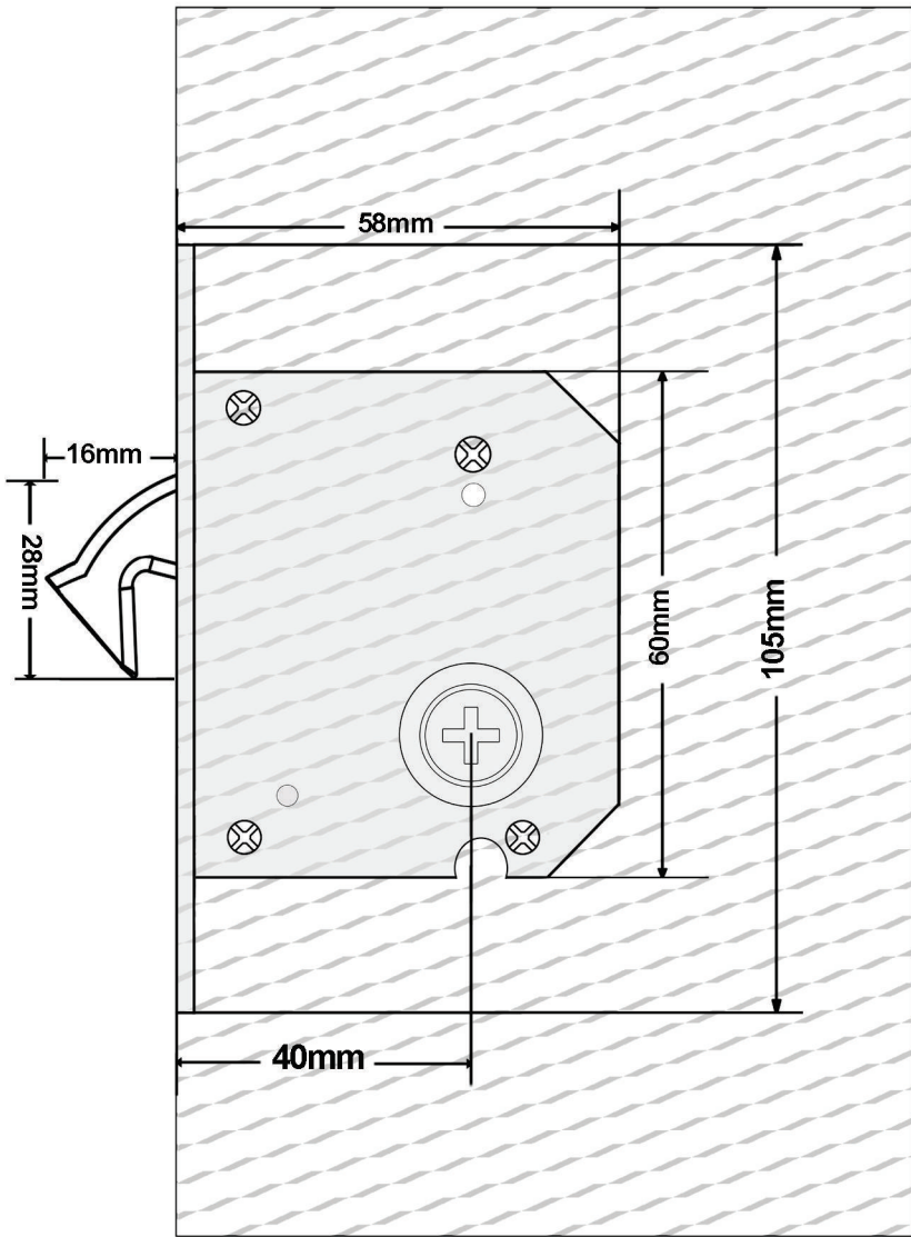
VISTA LATERAL DE LA CERRADURA, EN CORTE
